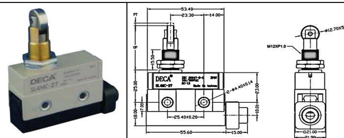
* SL4MC-27 面板安裝橫向滾輪、柱塞型
