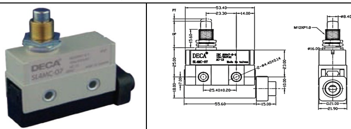
* SL4MC-07 面板安裝柱塞型
