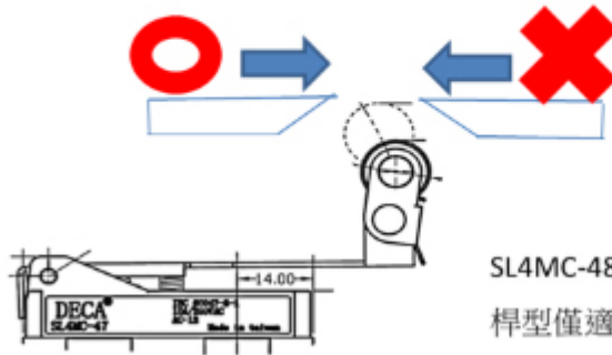
SL4MC-43 & SL4M-44 滾輪擺桿型可適用於雙向的檔塊
