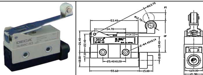
*SL4MC-43 臥式標準滾輪擺桿型
