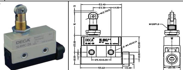
* SL4MC-26 面板安裝滾輪、柱塞型
